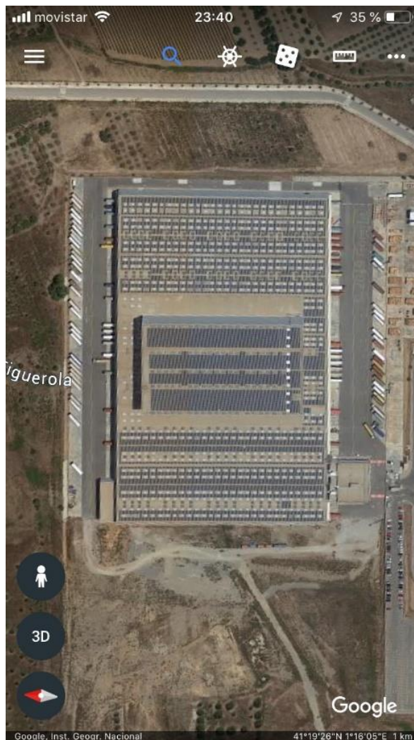
4,7MWp Mobles
